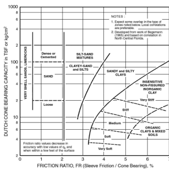
Gambar 1. Klasifikasi tanah berdasarkan Schmertmann, 1978
