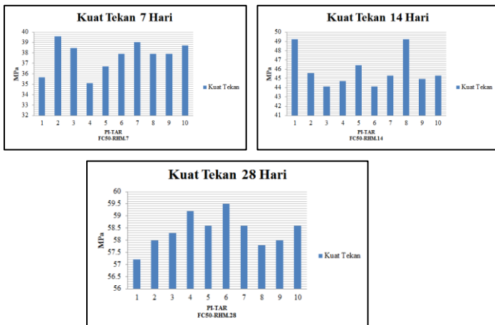
Gambar 3. Grafik Hasil Pengujian Kuat Tekan
